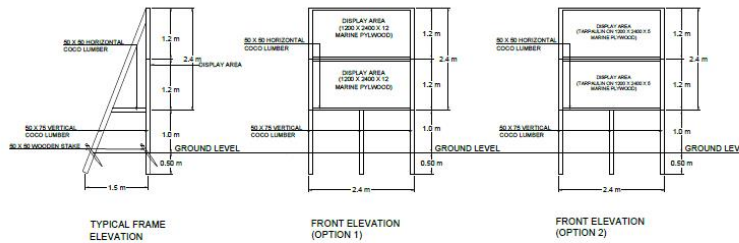
BILLBOARD FRAME SCALE: NTS
