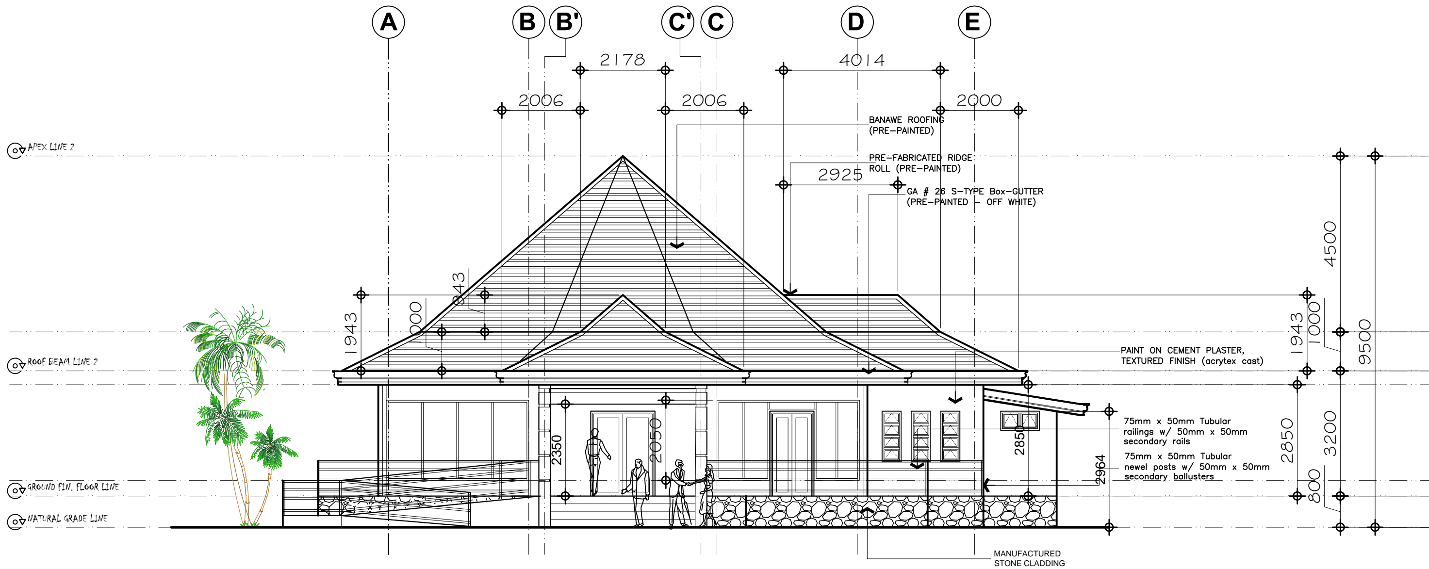
2 A 2 FRONT ELEVATION SCALE: 1:100
